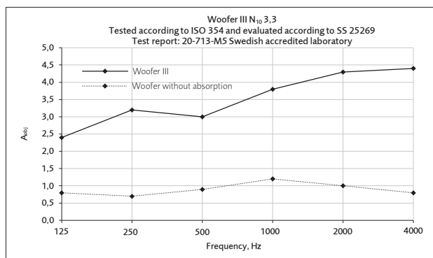
Ljudabsorptionsområde enligt ISO 354 och SS 25269
