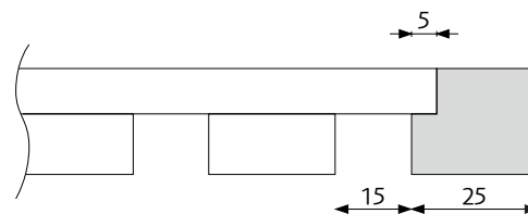
Kapad filt med avsltningslist
