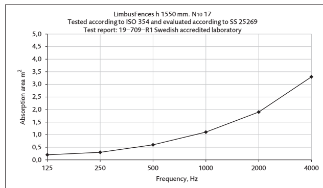
Ljudabsorptionsområde enligt ISO 354 och SS 25269
